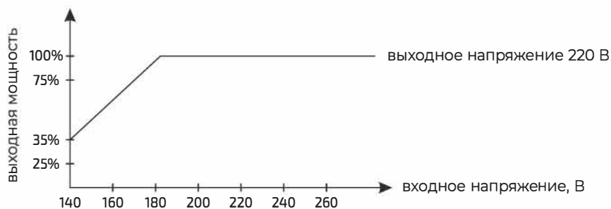
Рисунок 3. Нагрузочная характеристика
