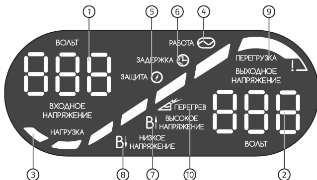
Рисунок 4. Элементы индикатора
