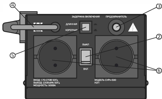
Рисунок 2. Вид сверху
